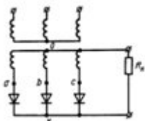
Б 2 - выпрямитель
